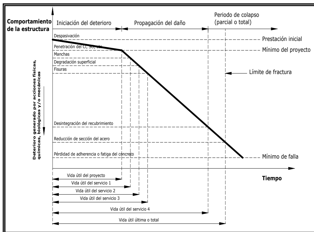
Figura 2: Comportamiento del concreto ante deterioro prolongado
